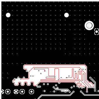
INNER LAYER
