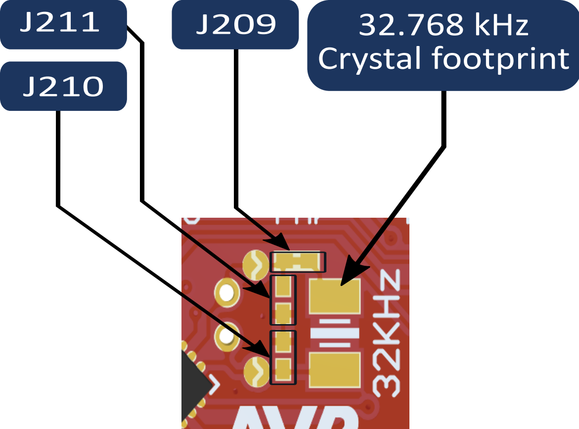
Top side
