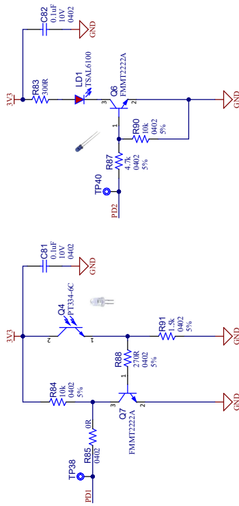
UART Opto-Port
